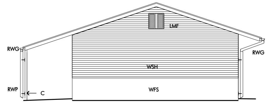
03 ELEVATION 3
