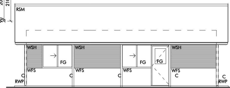
01 ELEVATION 1
